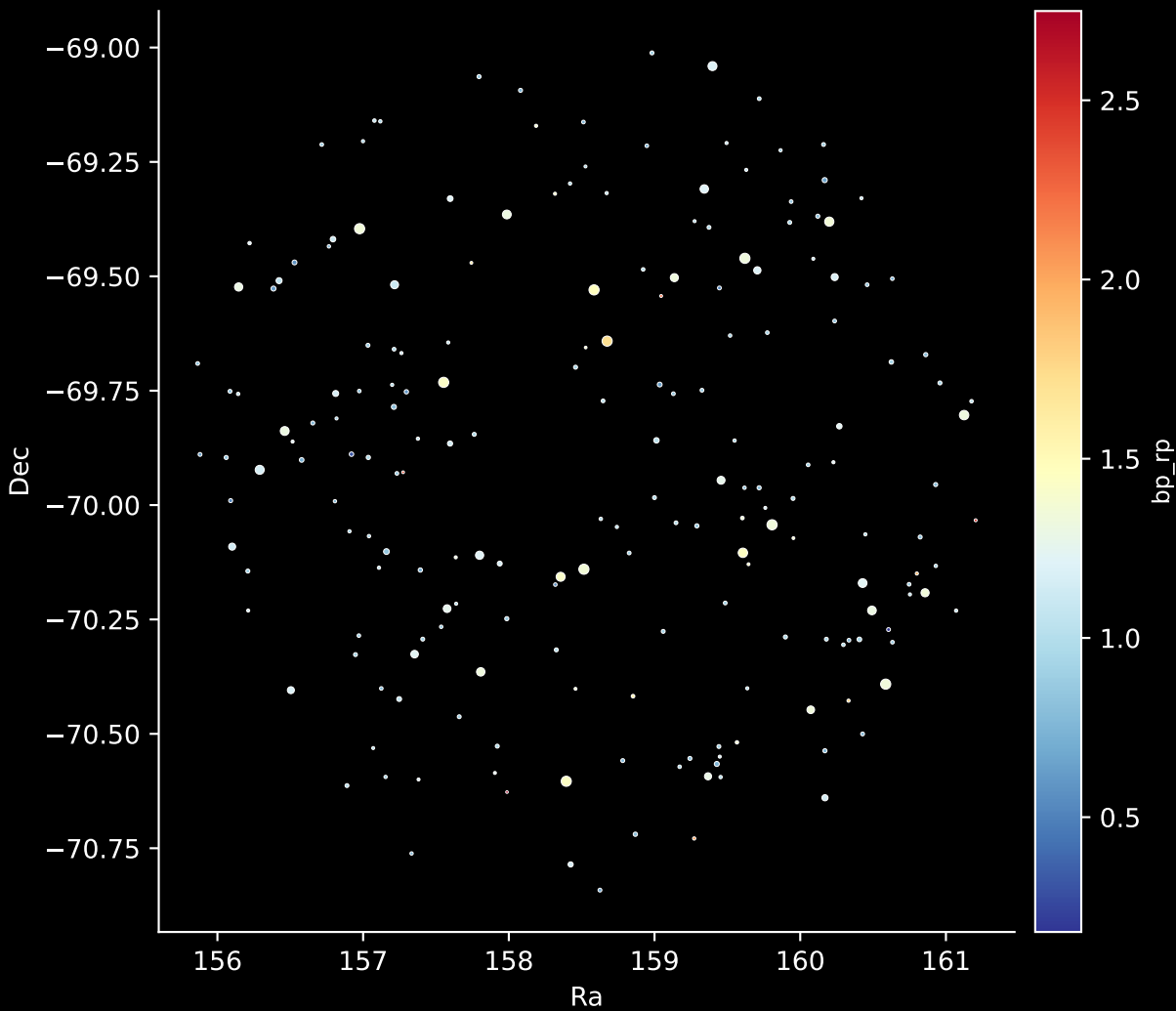
APOGEE DR17 Field: [284-40-O_TESS] Stars: 198
