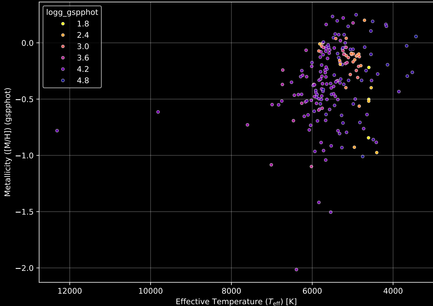
APOGEE DR17 Field: [284-40-O_TESS] Stellar Population Parameters (n= 198)
