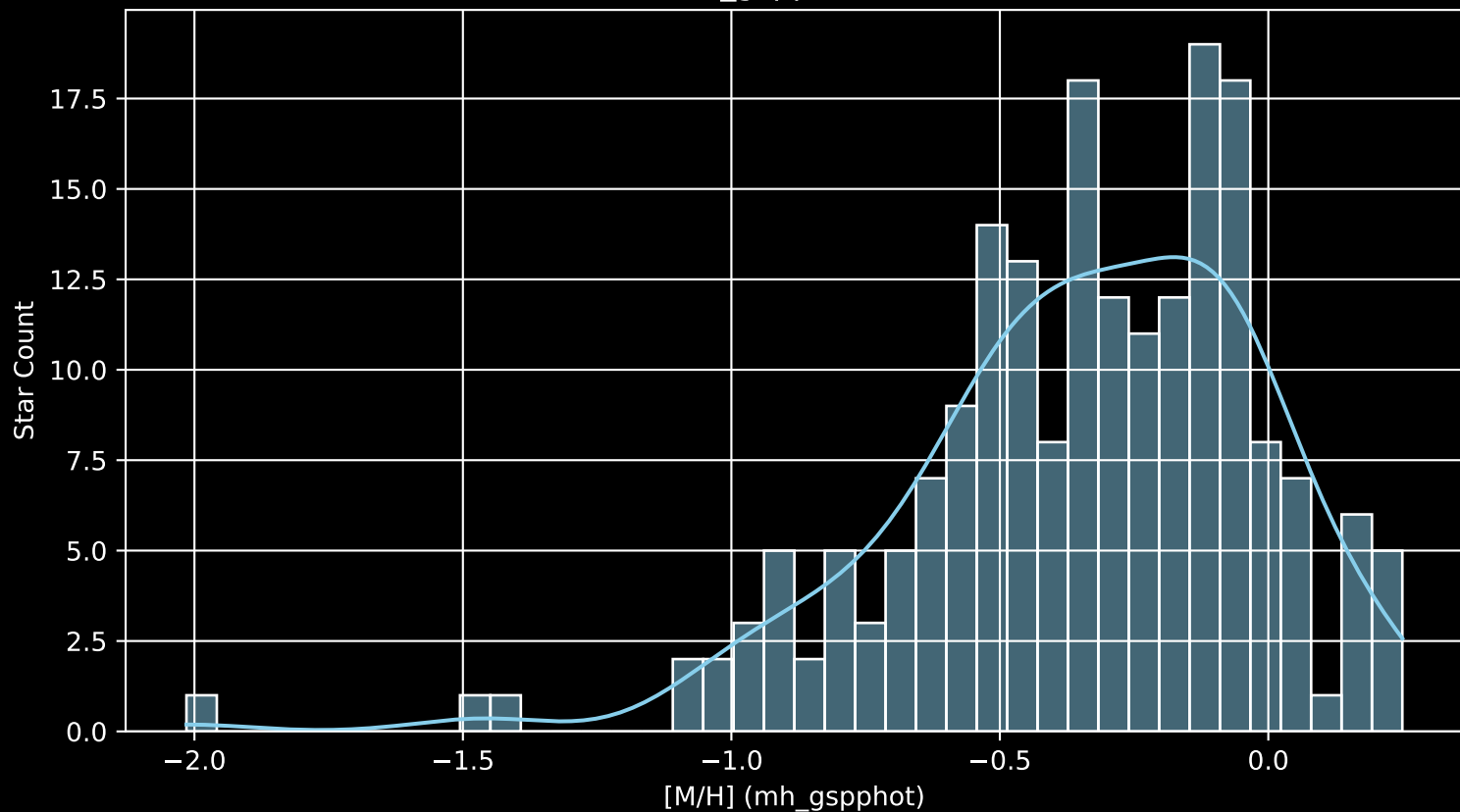
APOGEE DR17 Field: [284-40-O_TESS [M/H] (mh_gspphot) (n= 198)
